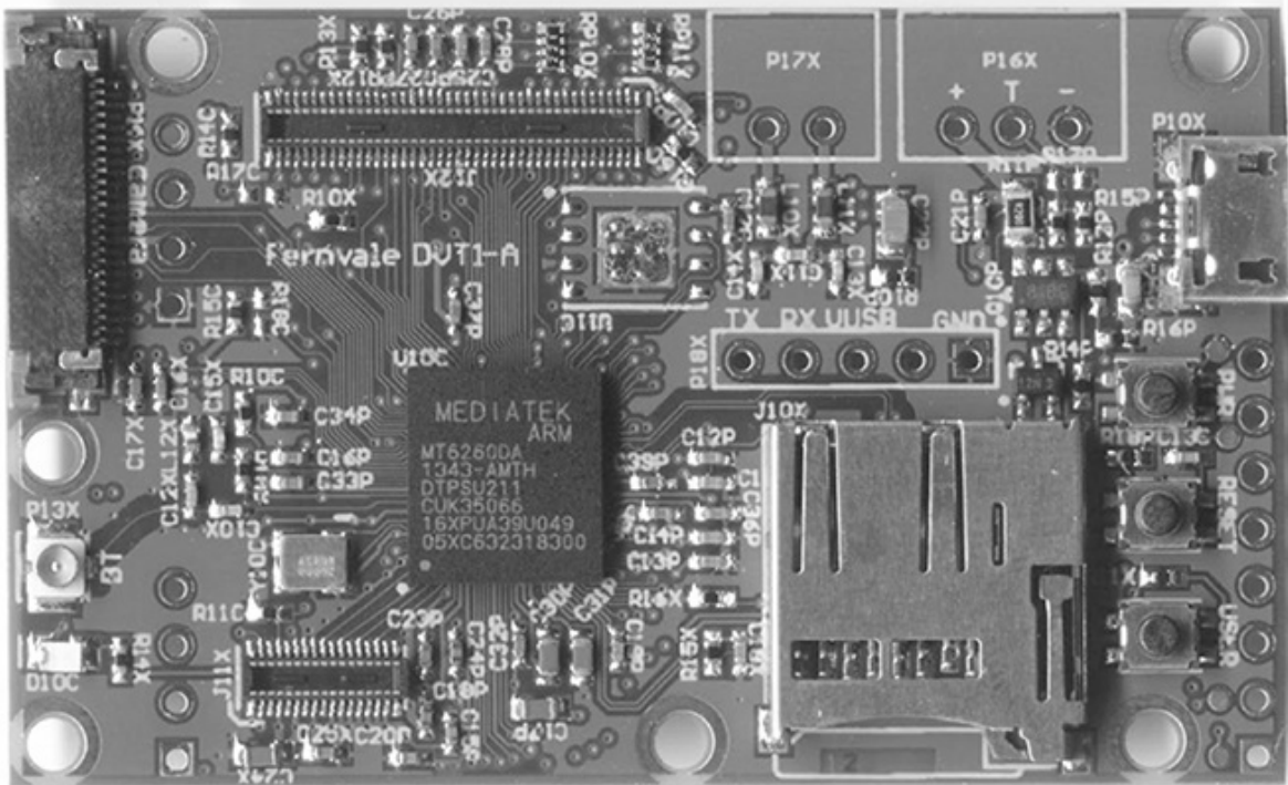
AFE header
