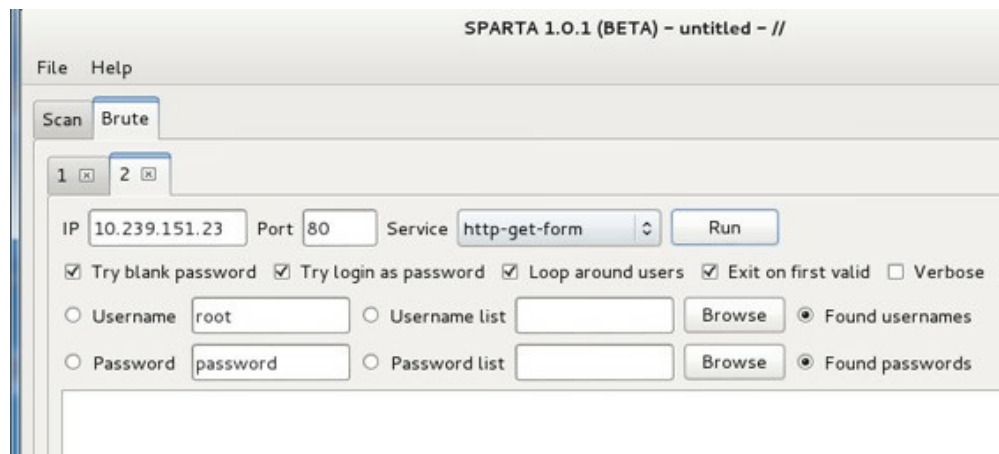
SPARTA - Brute
