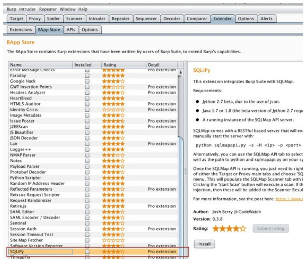
Burp - SQLiPy
