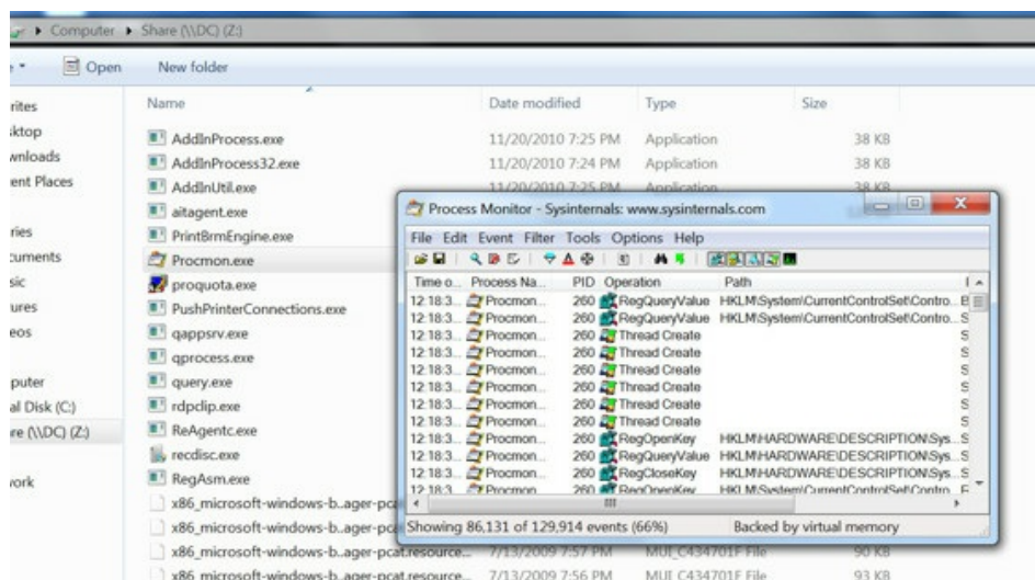
Malicious Procmon
