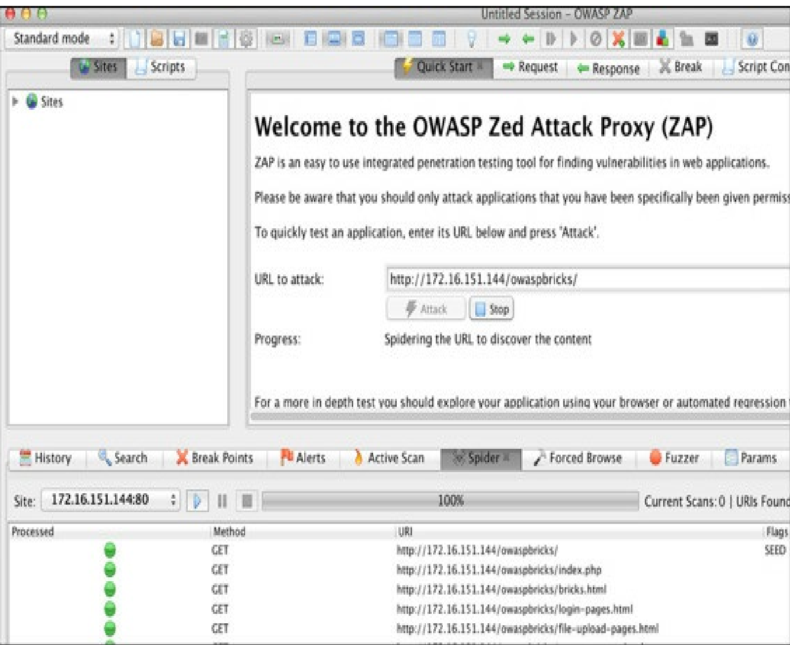
OWASP ZAP
