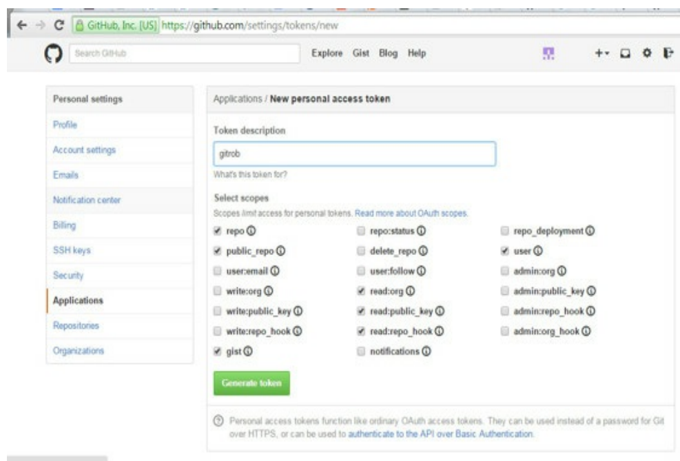
Gitrob search
